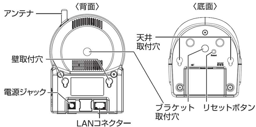
図 3-2 : 背面各部
