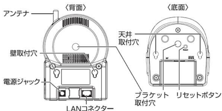
図 3-2：背面各部
