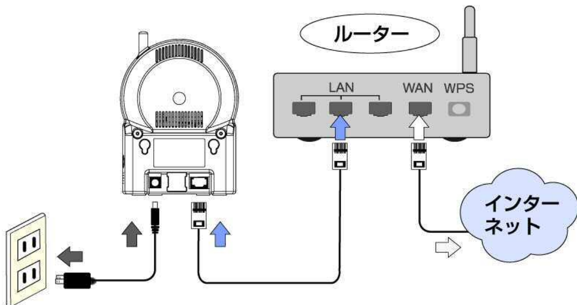
図 3-3 : IPC-07FHD 接続図
