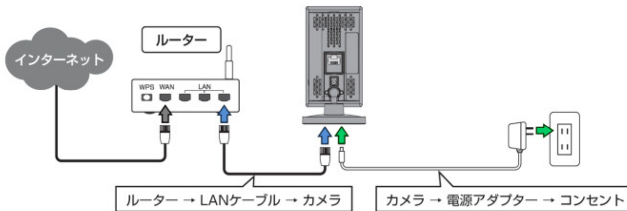
図 3-3 : IPC-09w 接続図
